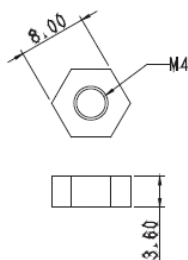
Écrou de verrouillage Plaque métallique B
